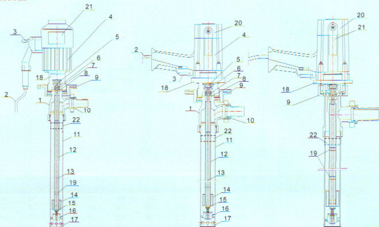
剖面图
